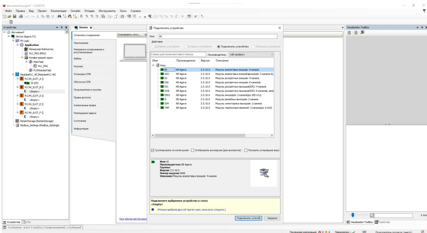
Рисунок 5-5. Подключение submodule
