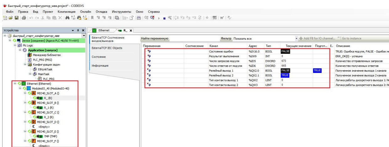
Рисунок 31. Выполнение проекта
