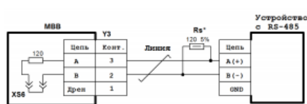
Схема подключения линии RS-485 к каналу 2 (Y3) (без дренажного провода)
