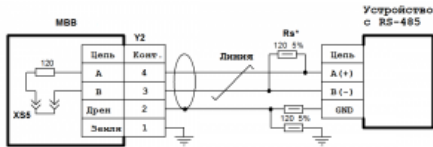
Схема подключения линии RS-485 к каналу 1 (Y2) (с дренажным проводом)
