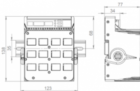
Габаритные размеры АГАВА МВВ-40
