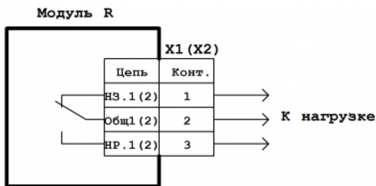
Схема подключения субмодуля дискретных выходов R
