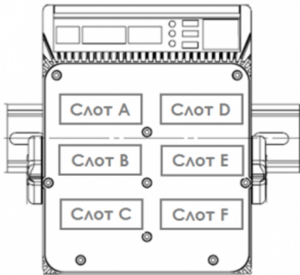
Расположение слотов для субмодулей
