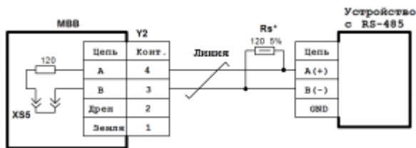
Схема подключения линии RS-485 к каналу 1 (Y2) (без дренажного провода)
