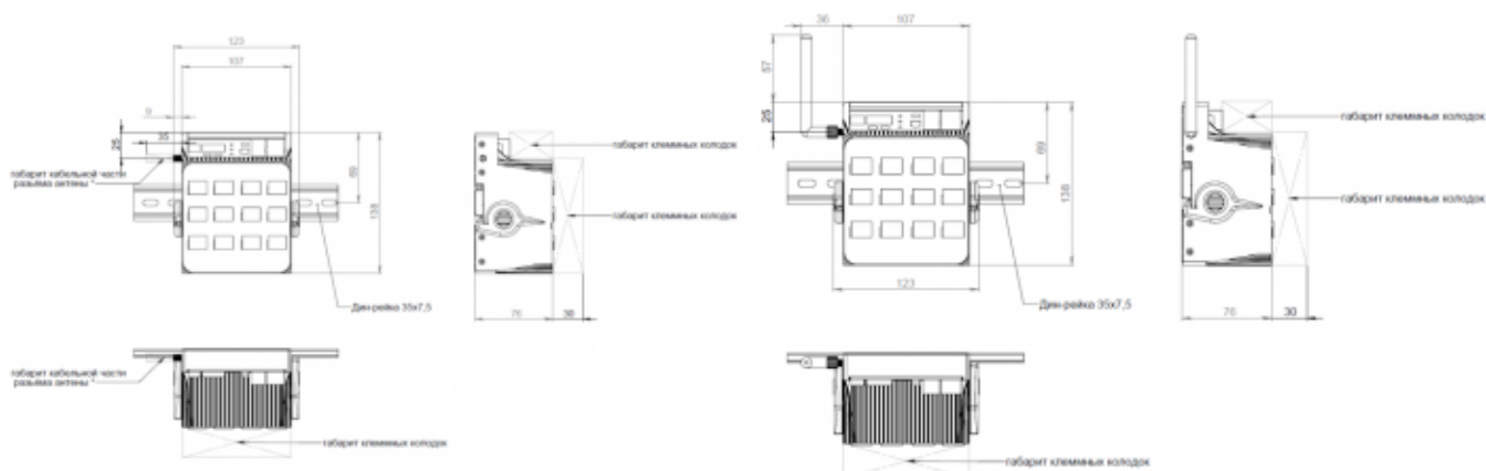
Габаритные размеры АГАВА МПР-60.WIFI с установленной антенной
