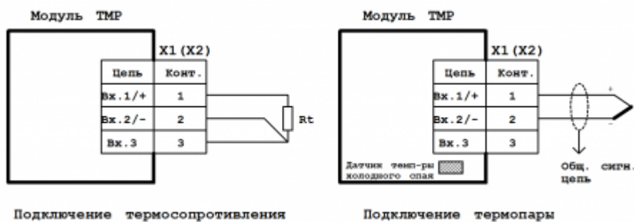
Подключение термосопротивления Подключение термопары Схема подключения субмодуля измерения температуры TMR
