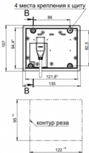
АГСФ.305413.003 Дисплей ПК-70 диагональ 4
