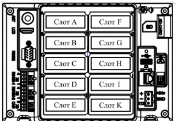
Расположение submodule
