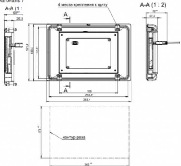
АГСФ.305413.004 Дисплей ПК-70 диагональ 10"
