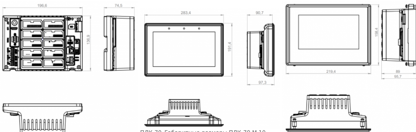
Габаритные размеры ПЛК-70.F
