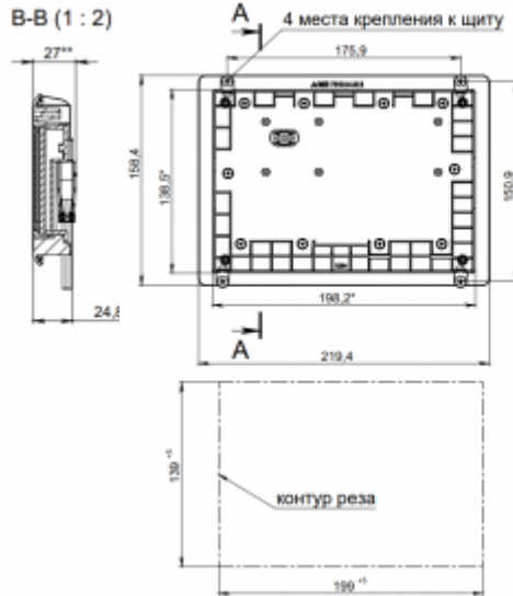
АГСФ.305413.001 Дисплей ПК-70 диагональ 7
