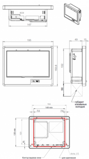
Габаритные размеры и размеры выреза в щите АГАВА ПО-50.07
