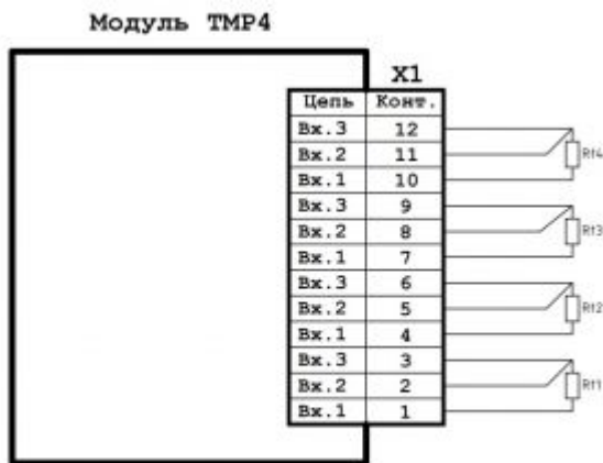
Подключение термосопротивлений
