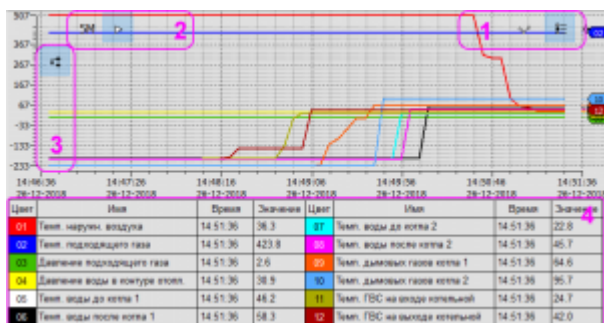
Рисунок 30 - Виджет «Исторический график». Области кнопок-пиктограмм. В нижней части отображена легенда
