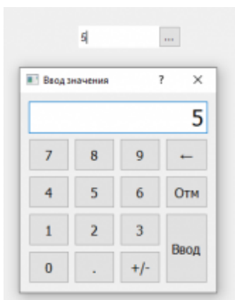
Рисунок 37 - Виджет
