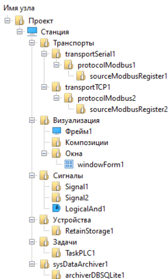
Рисунок 21 - Дерево проекта
