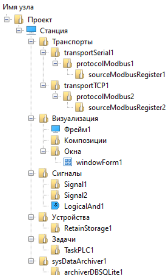
Рисунок 21 - Дерево проекта
