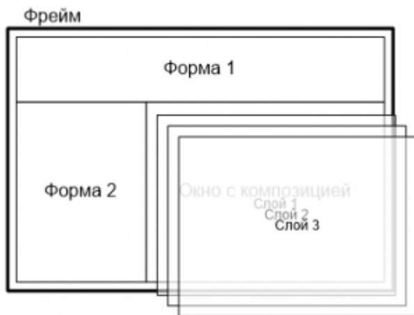
Рисунок 23 - Пример структуры сложного фрейма, состоящего из двух форм и одного окна с многослойной композицией
