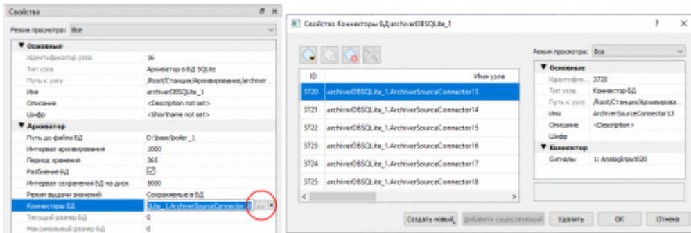
Настройка архиватора
