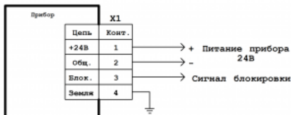
Схема подключения питания и сигнала блокировки к АГАВА МПР-60 ревизия 2
