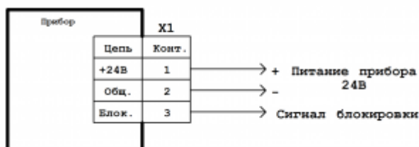
Схема подключения питания и сигнала блокировки к АГАВА МПР-60
