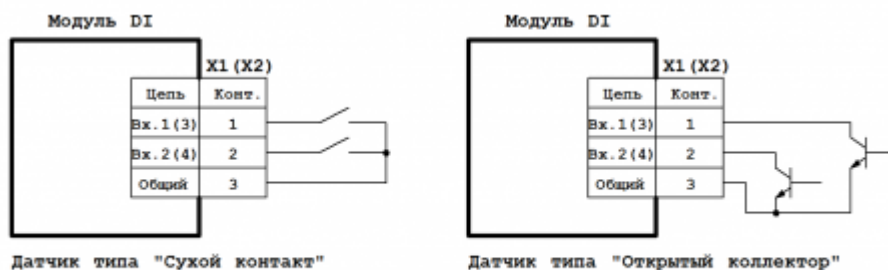
Датчик типа "Сухой контакт"
