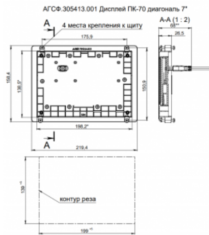
Размеры вырезов в щите ПК-70.7
