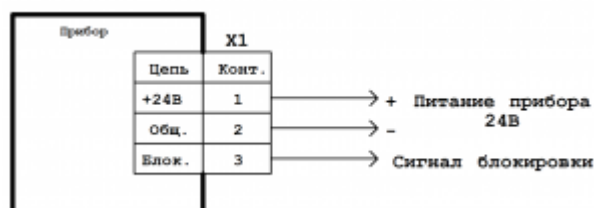
Схема подключения питания и сигнала блокировки к АГАВА ПЛК-70
