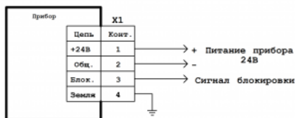
Схема подключения питания и сигнала блокировки к АГАВА ПЛК-70 ревизия 2
