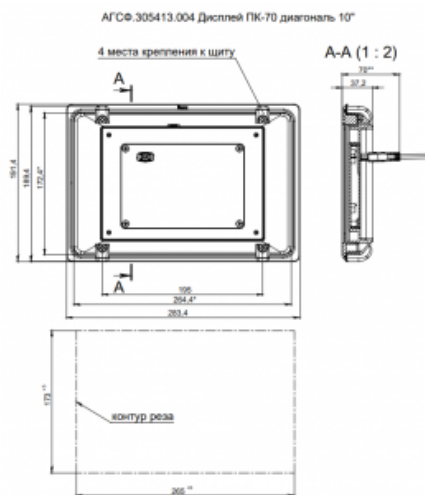
Размеры вырезов в щите ПК-70.10
